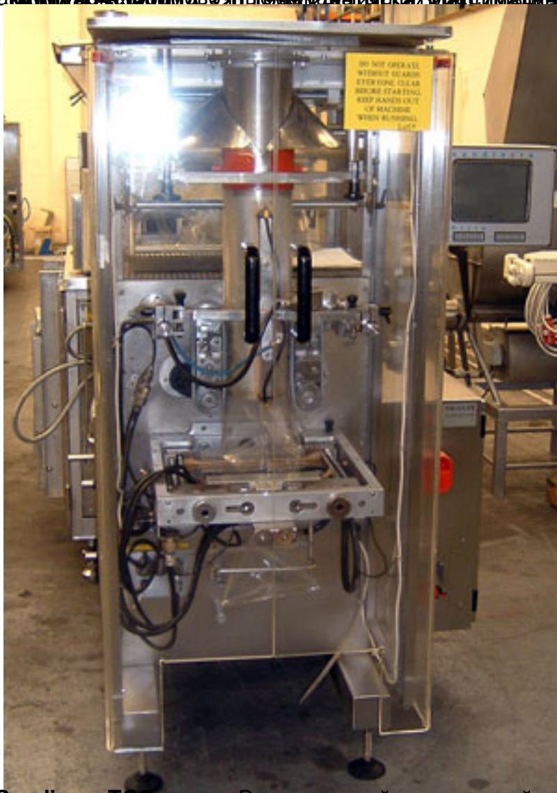
Sandiacre TG3. Вертикальный упаковочный автомат в формируемый из термосвариваемой пленки. Маркировочное оборудование.
